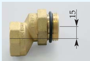
ART. 1513 Niplo disassato di 15 mm maschio/femmina M/F disassembled nipple (15 mm)
