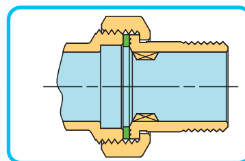
"CP": TENUTA CON GUARNIZIONE PIANA FLAT END WITH FLAT WASHER
